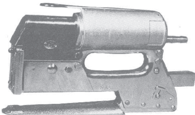
Paineil­makäyt­ttöinen yleis­ni­toja
