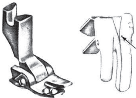
Paininjalka, langankatkaisulla
