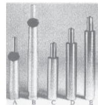
A Mekaaninen pystypilari (vakio) B Korkea mekaaninen pystypilari C Kaasujousi 140 mm (vakio) D Kaasujousi 200 mm E Kaasujousi 260 mm Korkeudet ilman pyöriä.
