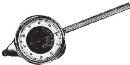
Kurvimittari (juoksumetrimittari).
