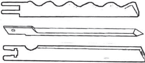
Pystyteräleikkurinteriä tyyppi HSS
