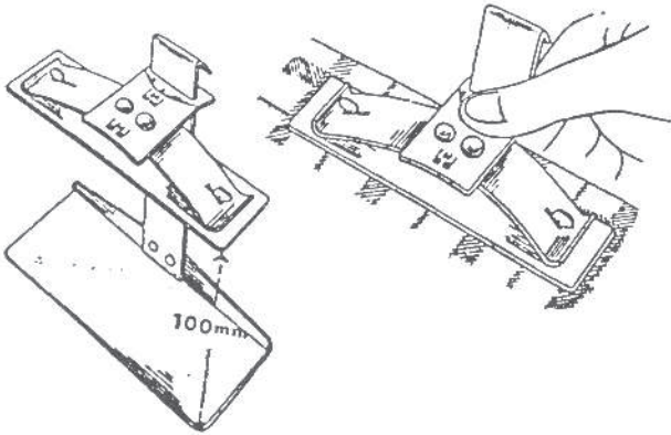
Levyllä varustettu jousipuristin, 100 mm
